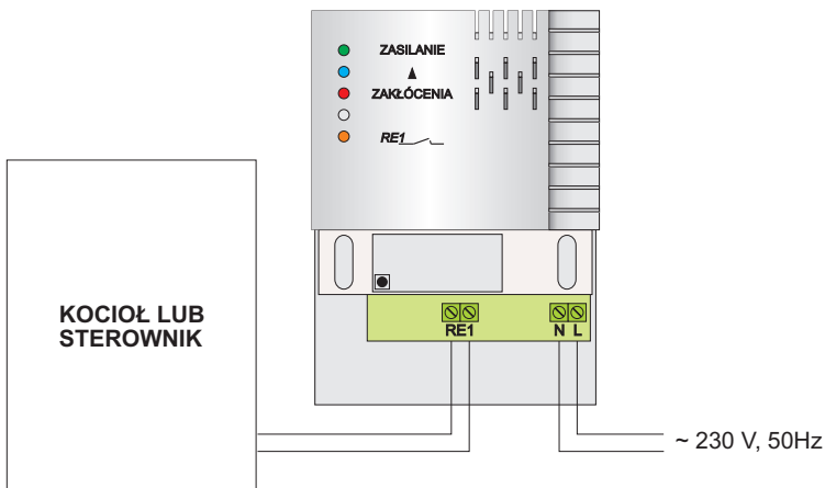
Rys. 4 Schemat podłączenia odbiornika do kotła / sterownika i do instalacji elektrycznej
